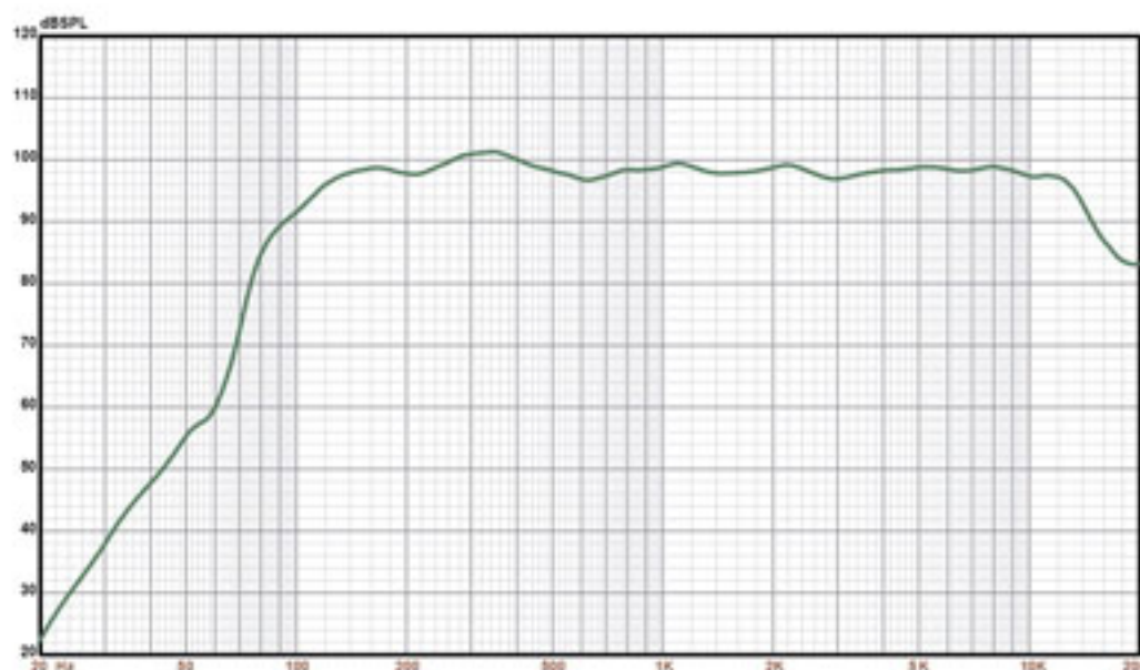
Curva de resposta em frequência, do sistema NBA45FR = BEYMA depois de inserido, o gerenciamento digital externo.
